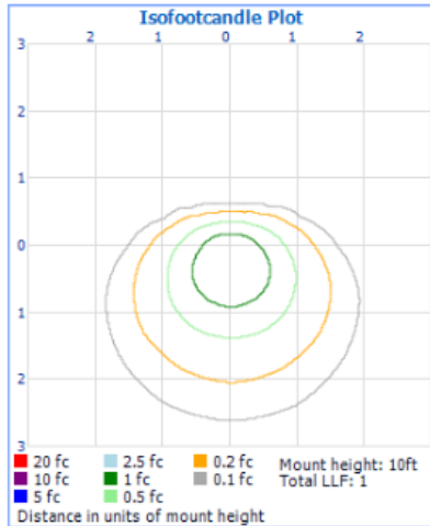
Isofootcandle Plot
